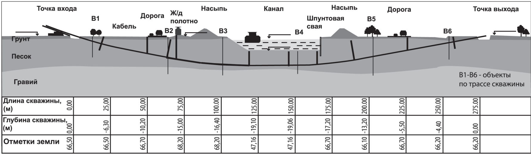
План
