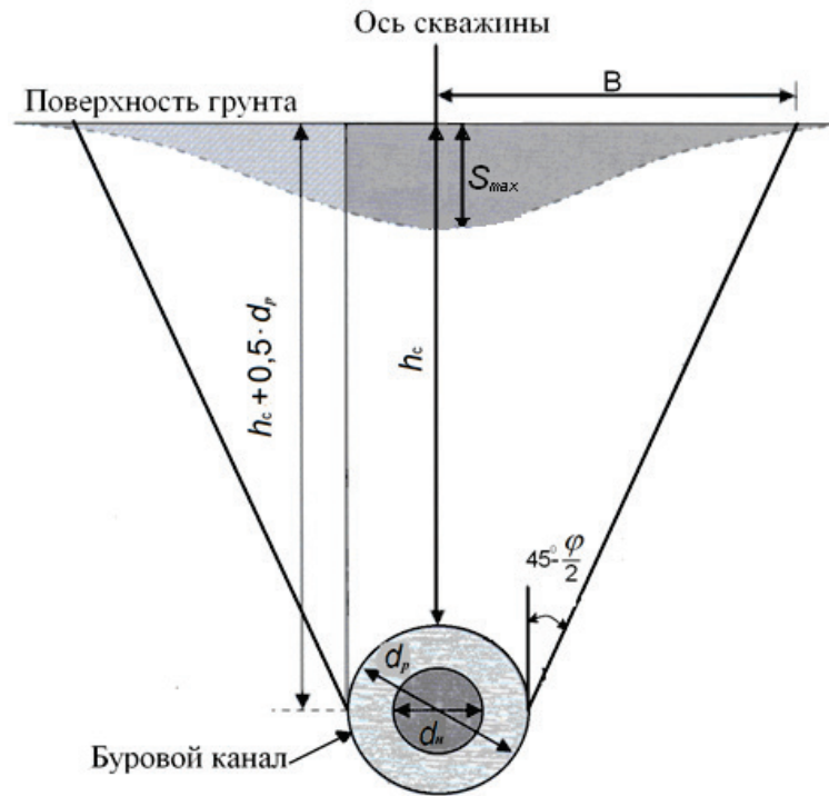
Рисунок 7.2 – Распределение осадок поверхности для скважин ГНБ
