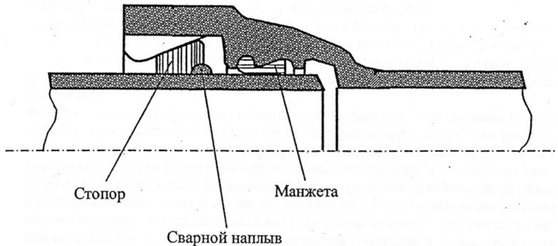
Рисунок 7.3 – Разрез раструбно-замкового соединения
