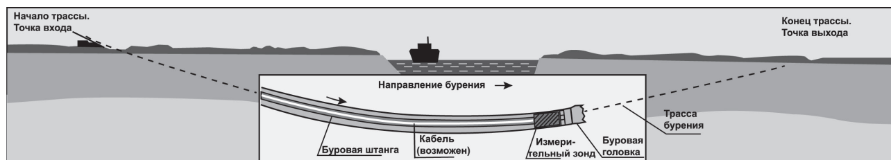
Рисунок 8.3 – Направленное бурение пилотной скважины
