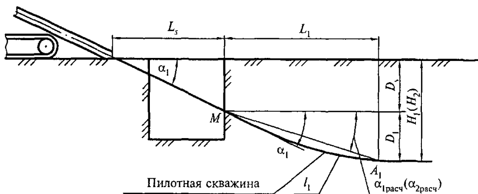
Рисунок Г.2 - Схема забуривания пилотной скважины.
