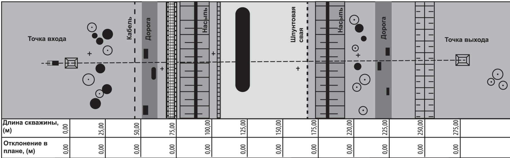
Рисунок А.1– Схема продольного профиля и плана закрытого подземного перехода, сооружаемого методом ГНБ
