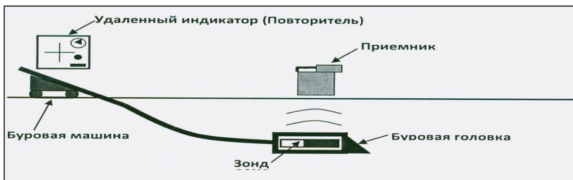
Рисунок Д.2 – Схема действия электромагнитной системы подземной локации
