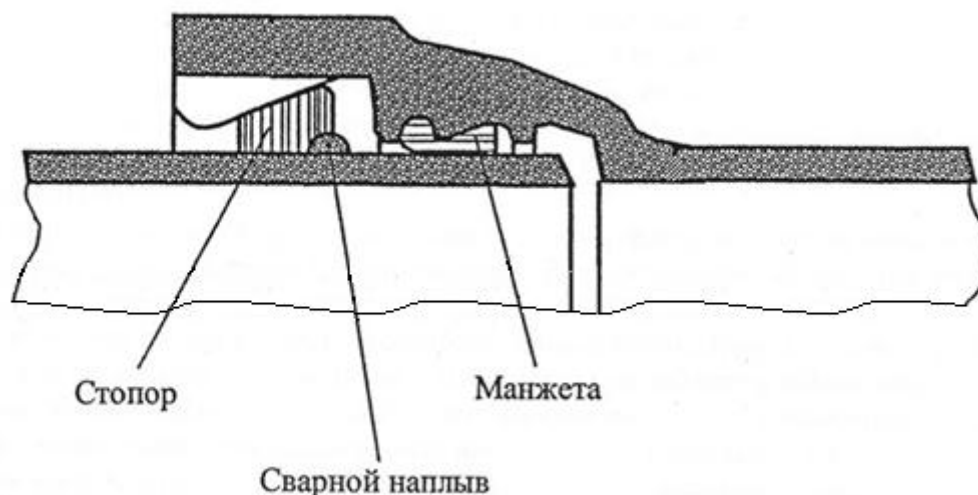
Рисунок 7.4 – Разрез раструбно-замкового соединения
