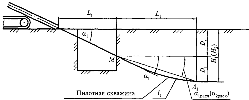
Рисунок Г.2 - Схема забуривания пилотной скважины.
